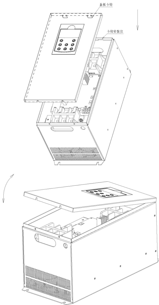
图3-2 上盖板拆卸图
