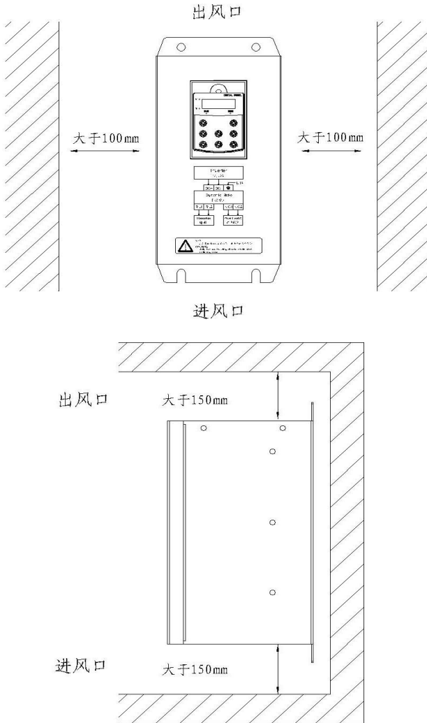
图 3-1 单体安装图
