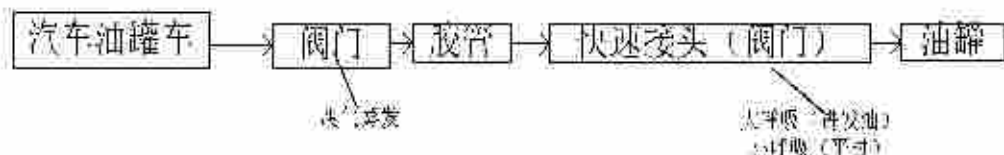
图 3-6 柴油油罐车装卸工艺流程图
