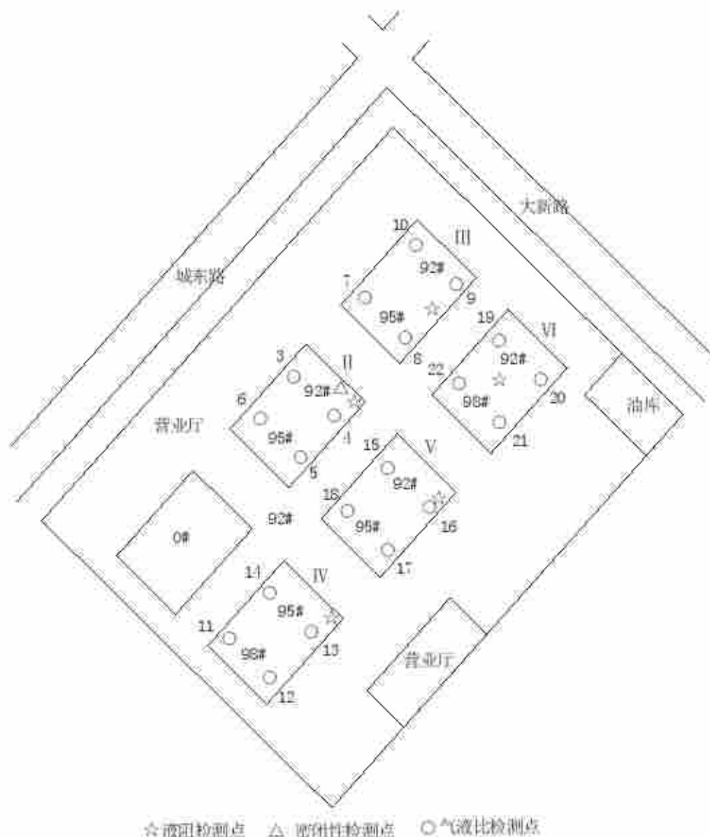
图 9-1 气液比、密闭性、液阻监测点位
