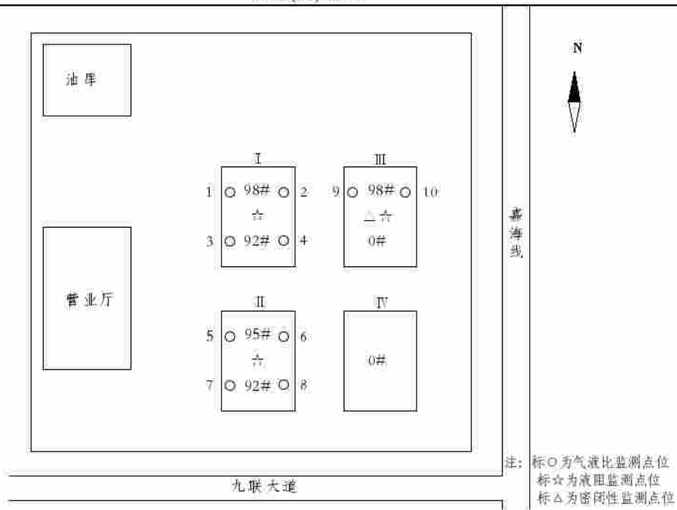
图 3-3 油气回收监测平面布置图
