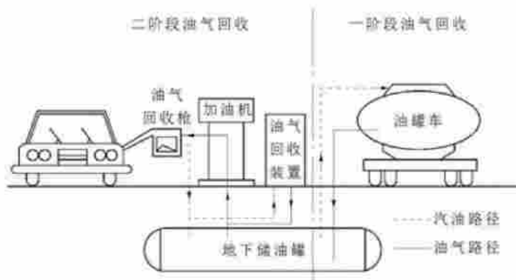
图 4-2 油气回收实施方案原理图
