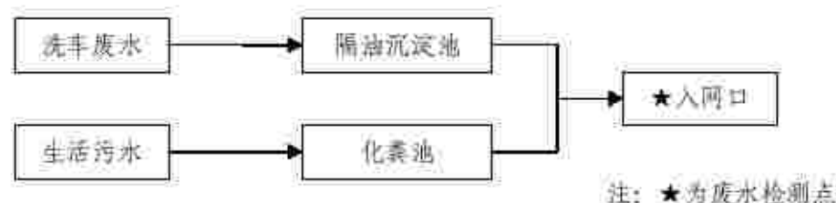
图 4-1 废水处理工艺流程
