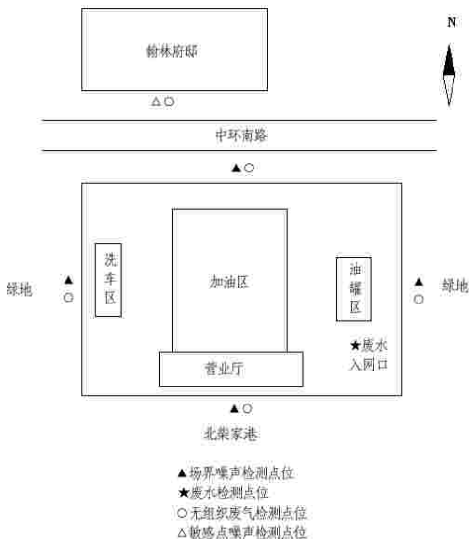
图 3-2 项目平面布置图
