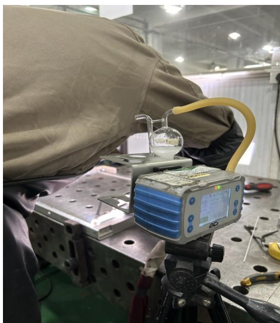
生产车间氩气焊岗位
