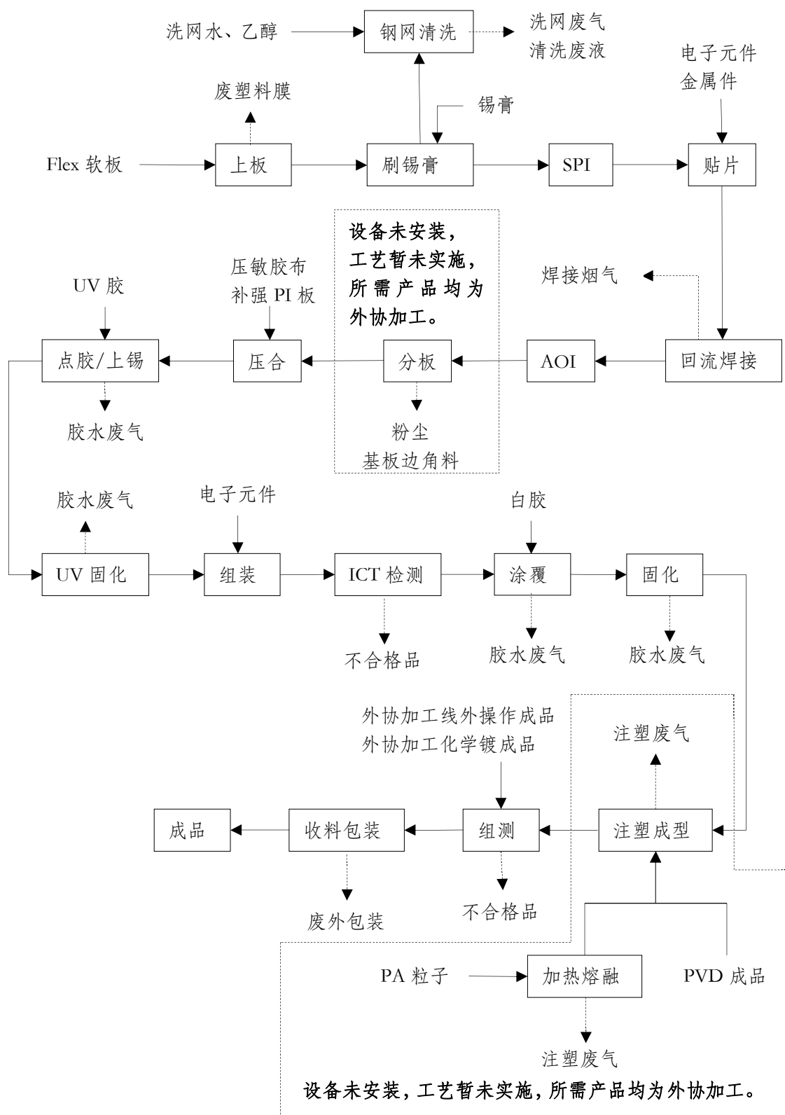
图 3-4 SMT 生产工艺流程图
