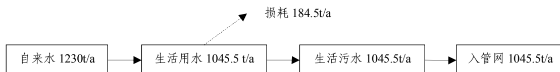
图 3-3 已建项目水平衡图
