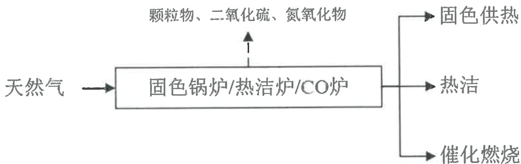
图 3-3 生产工艺及产污流程图
