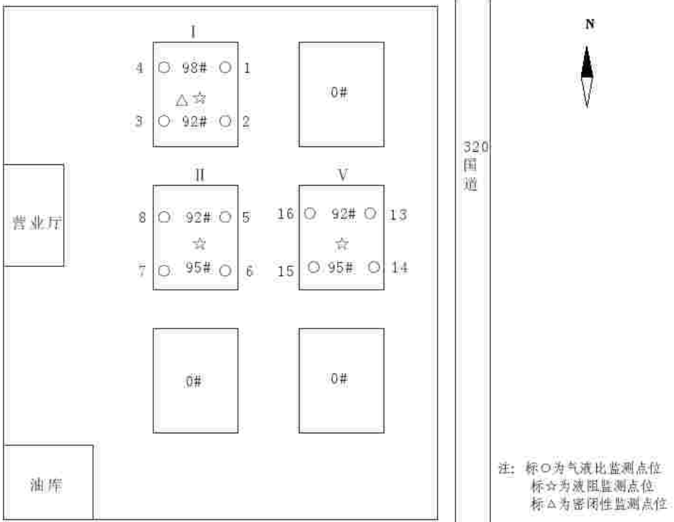
图 3-3 油气回收监测平面布置图
