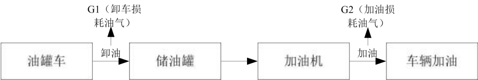
图 3-4 柴油生产工艺流程及产污环节
