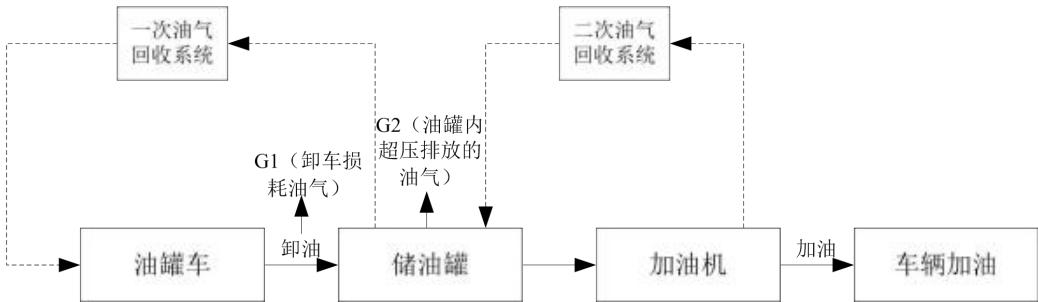
图 3-5 汽油生产工艺流程及产污环节
