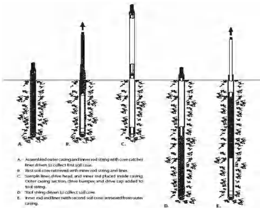
图 9-2 采样示意图
