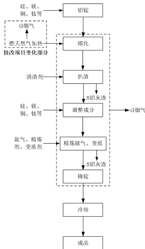
图 4-9 铝合金锭生产工艺流程图
