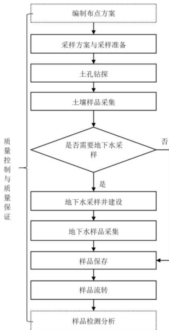
图 3-2 疑似污染地块现场采样工作程序
