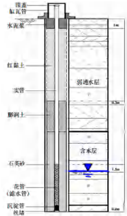
图 9-5 地下水监测井结构示意图
