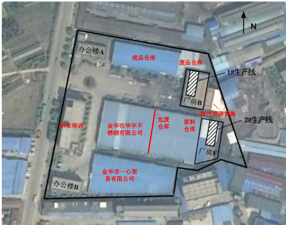
图 4-7 企业平面布置图
