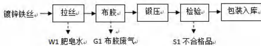
图 2 订书针生产工艺及产污流程图
