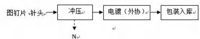
图 3-7 图钉生产工艺及产污流程图
