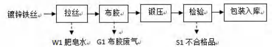
图 3-5 订书针生产工艺及产污流程图
