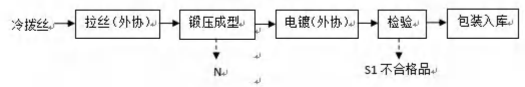
图 3-4 回形针、大头针生产工艺及产污流程图
