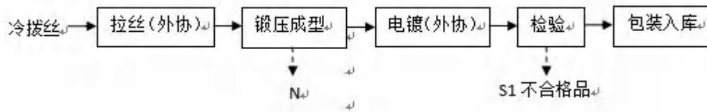
图 1 回形针、大头针生产工艺及产污流程图
