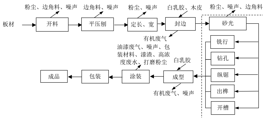
图 3-4 项目主要生产工艺及产污流程图
