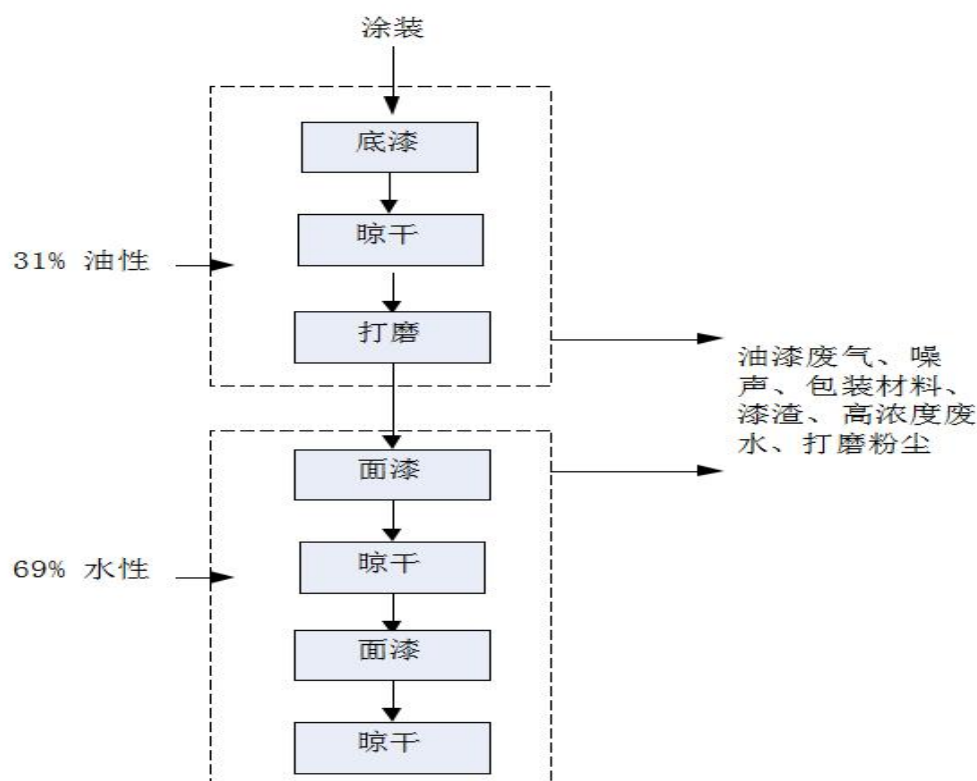
图 3-5 项目涂装工艺及产污流程图
