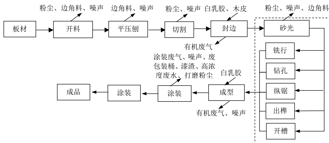
图 3-4 项目主要生产工艺及产污流程图
