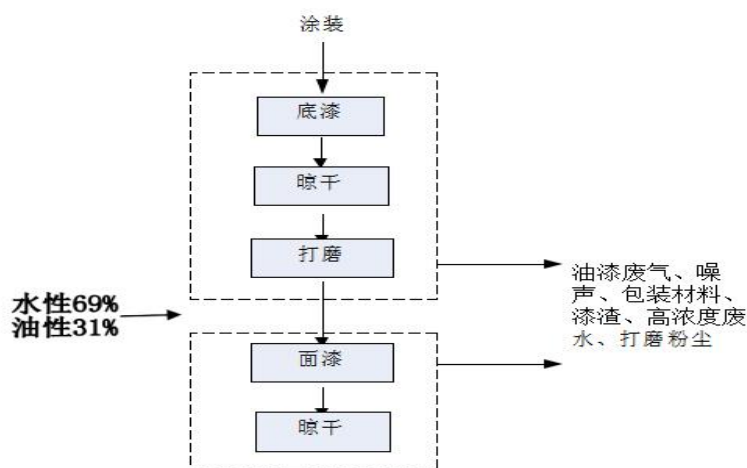
图 3-5 项目涂装工艺及产污流程图
