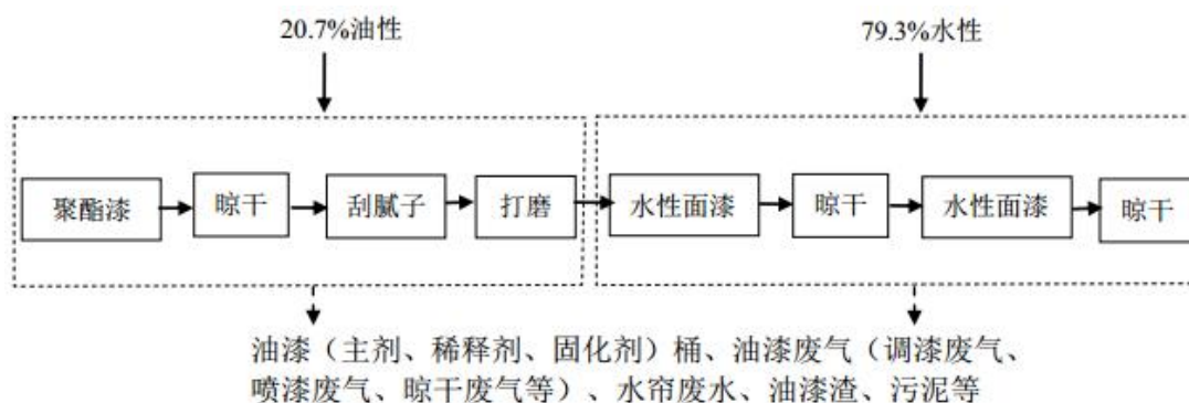
图 3-5 项目涂装流程及产污环节图
