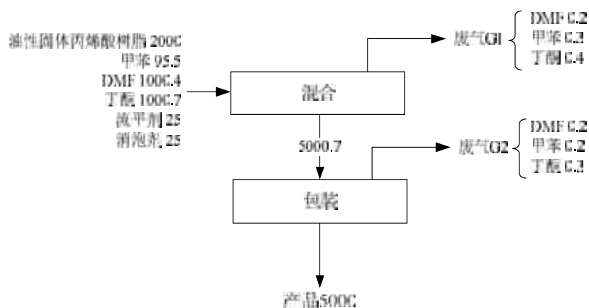
图3-11 油性丙烯酸树脂生产工艺流程图
