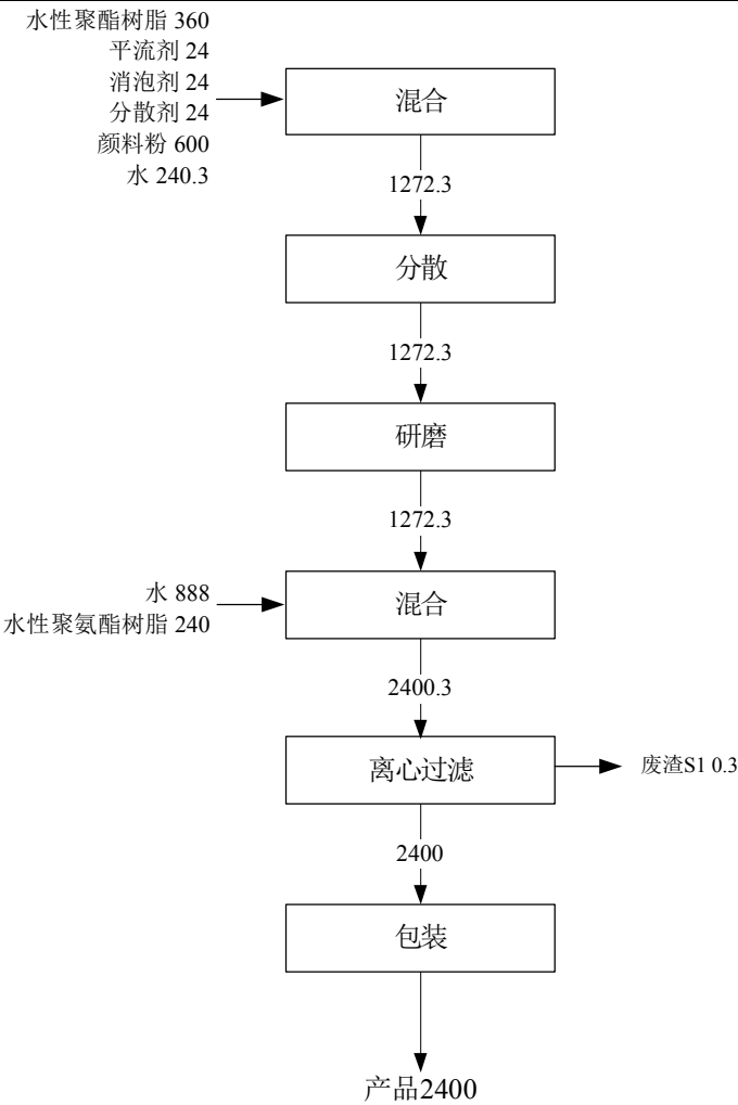
图3-7 水性色浆生产工艺流程图
