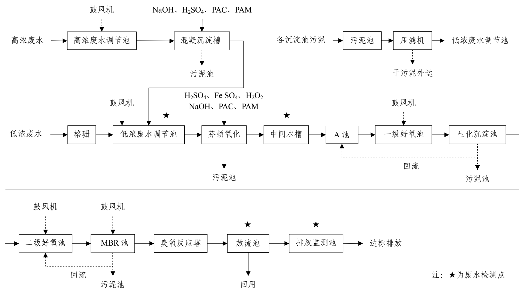
图 4-1 废水处理工艺流程
