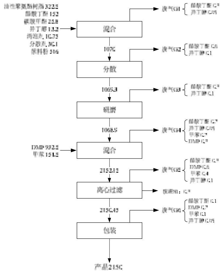
图3-6 低浓度油性色浆生产工艺流程图
