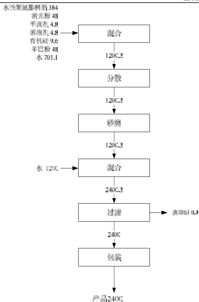
图 3-4 水性表面处理剂生产工艺流程图
