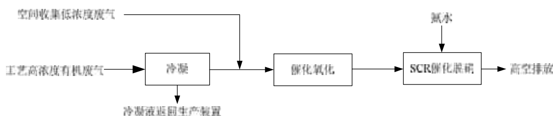
图3-14 环评设计有机废气处理工艺
