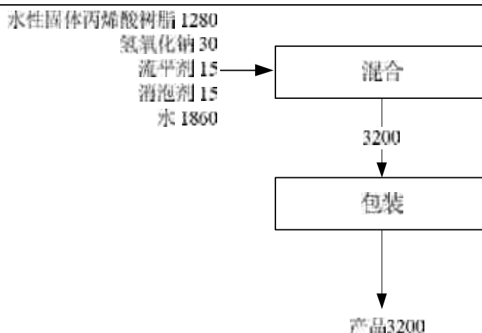
图3-10 水性丙烯酸树脂生产工艺流程图
