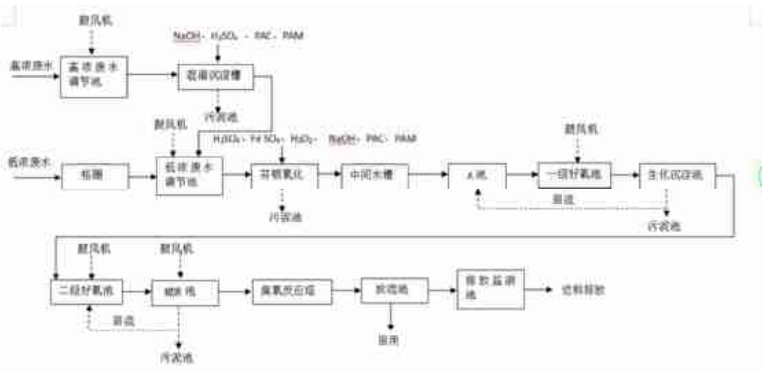
图3-13 实际建设污水处理工艺
