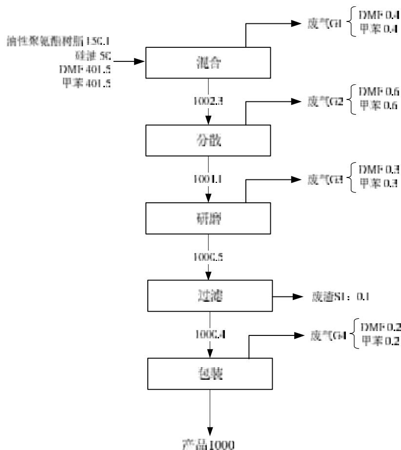
图3-8 油性助剂生产工艺流程图
