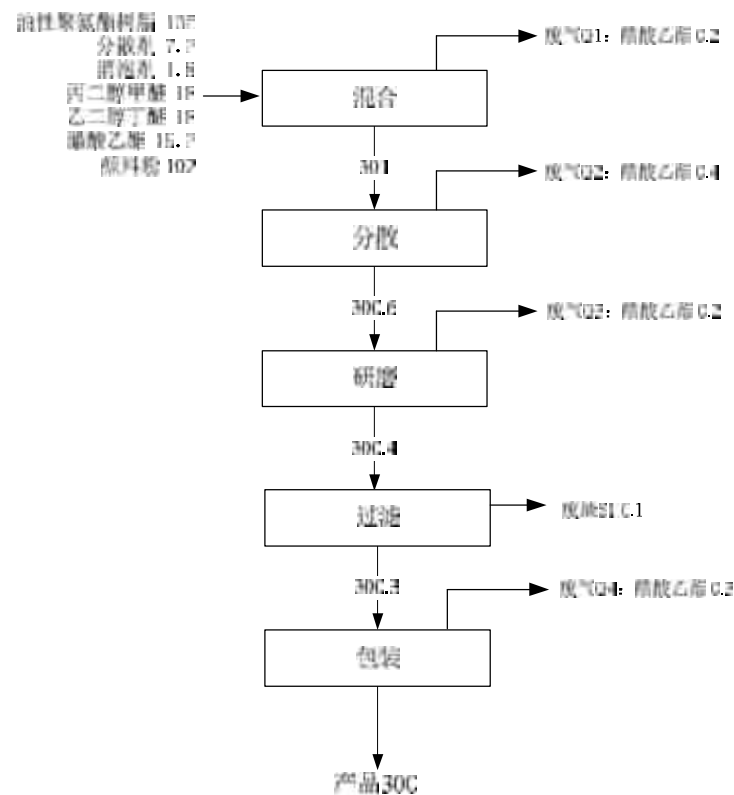
图 3-5 高粘度油性色浆生产工艺流程图
