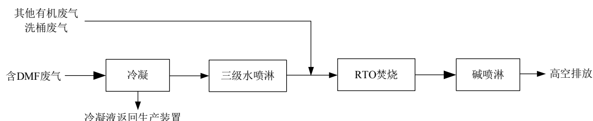
图3-15 实际建设有机废气处理工艺
