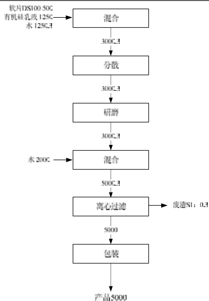
图3-9 水性助剂生产工艺流程图
