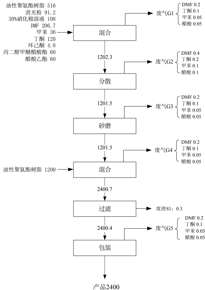
图 3-3 油性表面处理剂生产工艺及产污流程图
